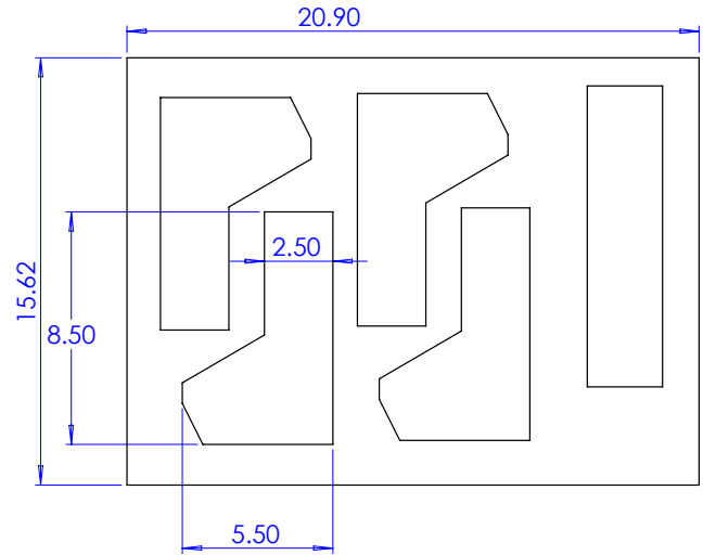
TOP LAYER
